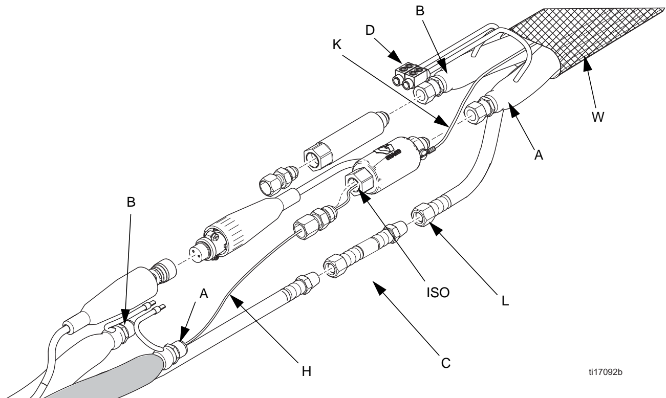
FIG. 9. Sensor de temperatura del fluido y mangueras calefaccionadas
