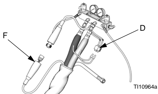
FIG. 8. Manguera calentada
